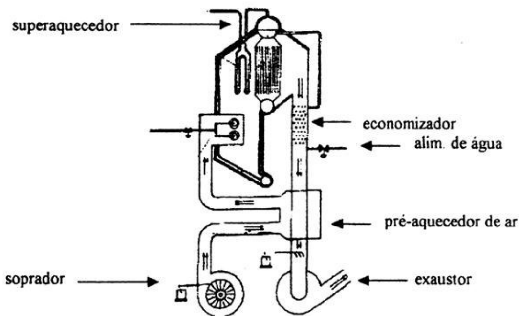
Figura 16 - Caldeira Aqua-tubular
