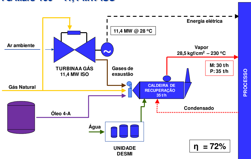
Figura 20 - Configuração com Turbina Mars 100
