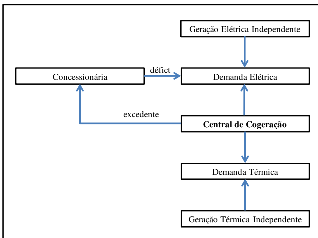
Figura 3 - Esquema básico de atendimento de demandas de energia (Balestieri 2002)
