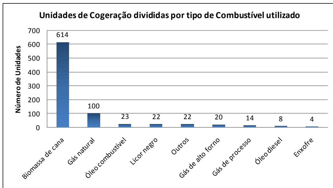
Gráfico 4 - Unidades de Cogeração, por tipo de combustível utilizado (Cogem/SP)
